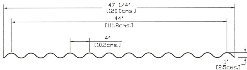
Acanalado 35 Tipo Rural
