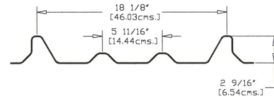
Acanalado 29 Tipo KR-18
