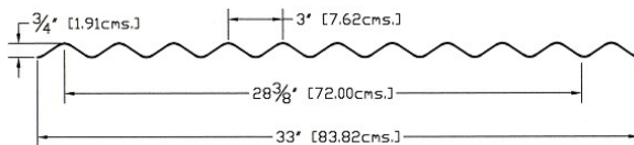
Acanalado 3 Tipo OI-30
