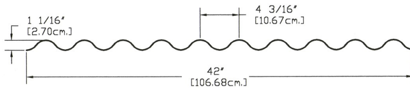
Acanalado 23 Tipo OT-42
