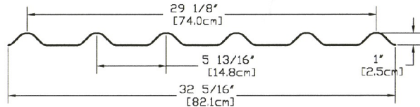
Acanalado 8 Tipo RG-74
