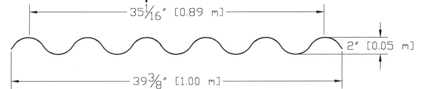
Acanalado 16 Tipo OA-100
