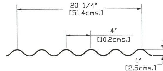
Acanalado 36 Tipo Rural de 60cms
